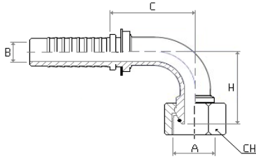
IPN40
